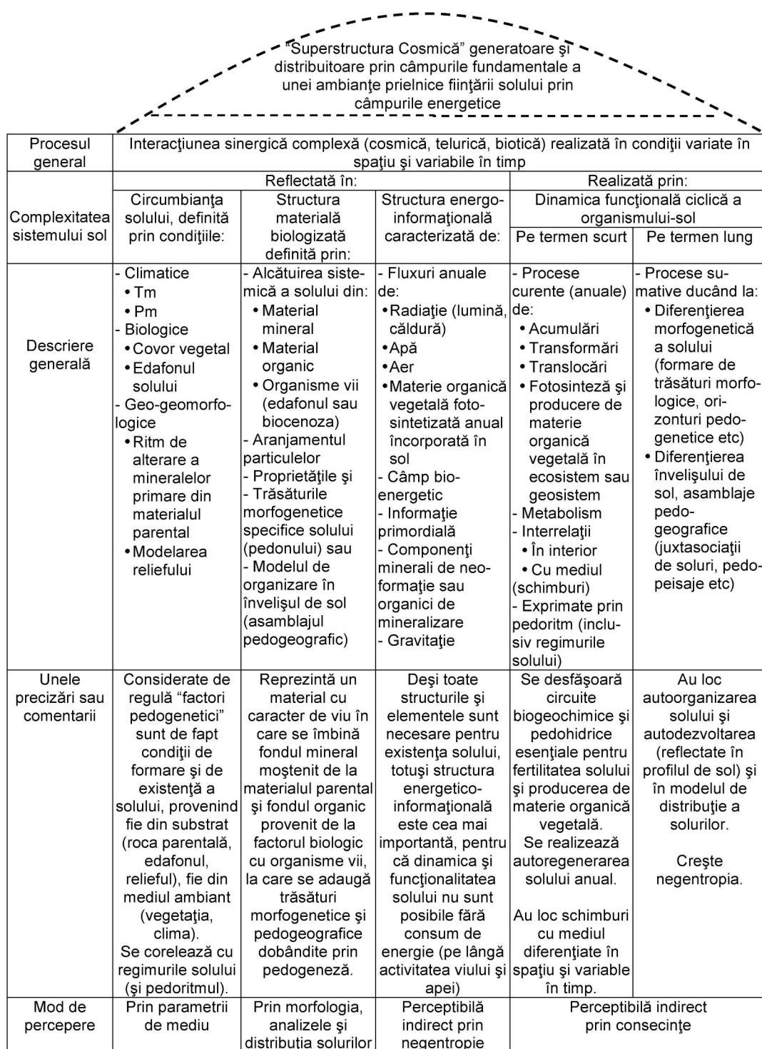
Fig. 1 Complexitatea, coerența și dinamica organismului-sol în natură (component esențial în ecosistem, geosistem). Superstructura Cosmică reprezintă, prin câmpurile energo-informaționale fundamentale, sursa fluxurilor de energie, informație și substanțe implicate în dinamica solului (formare, dezvoltare, evoluție).
